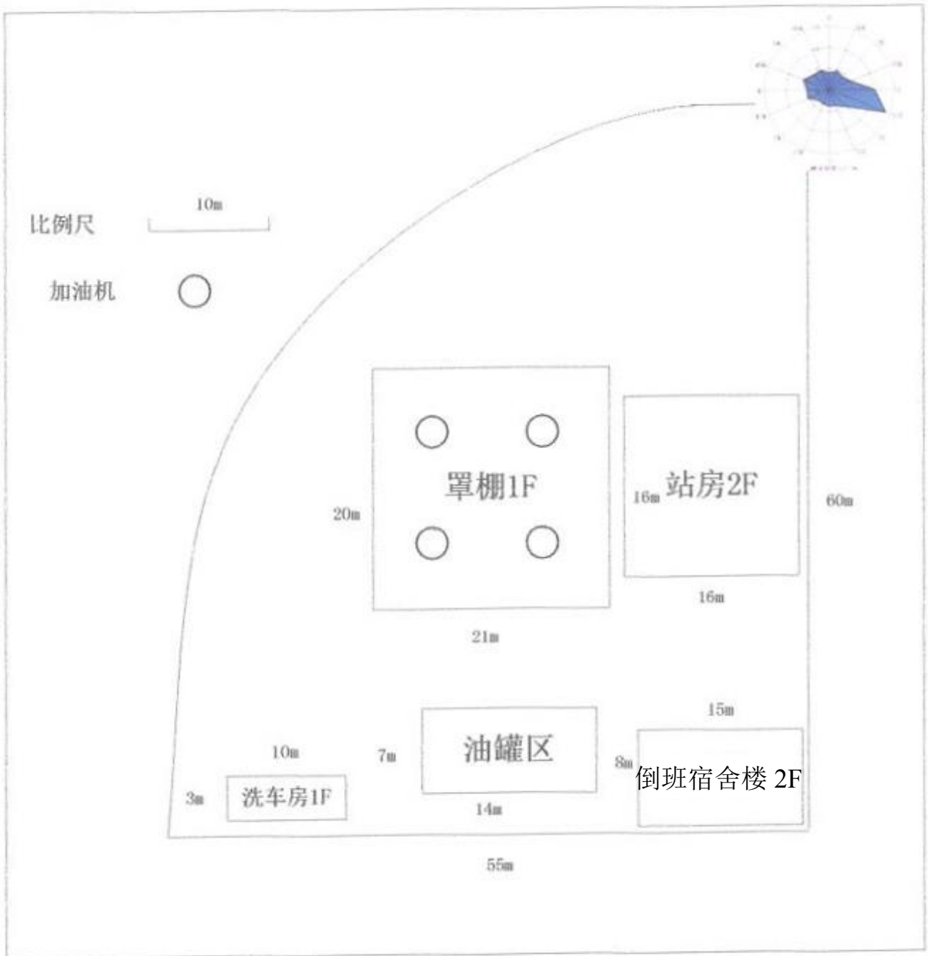
附图 4 厂区平面布置图
