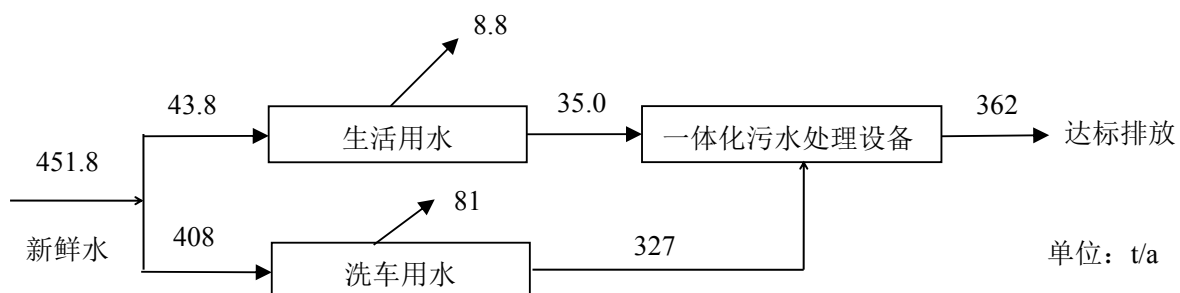
图 3-1 本项目水平衡图
