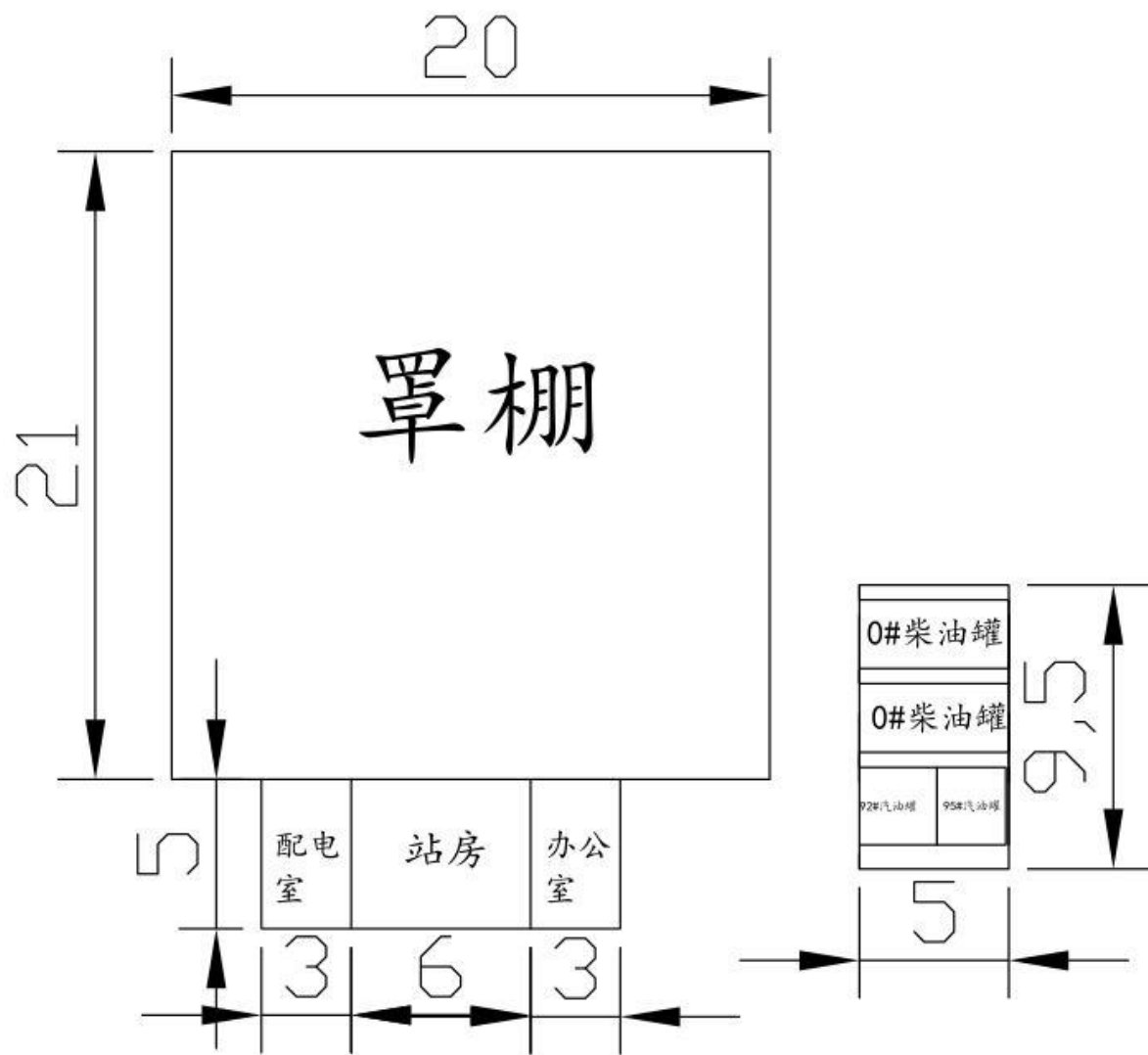
附图 4 厂区平面布置图
