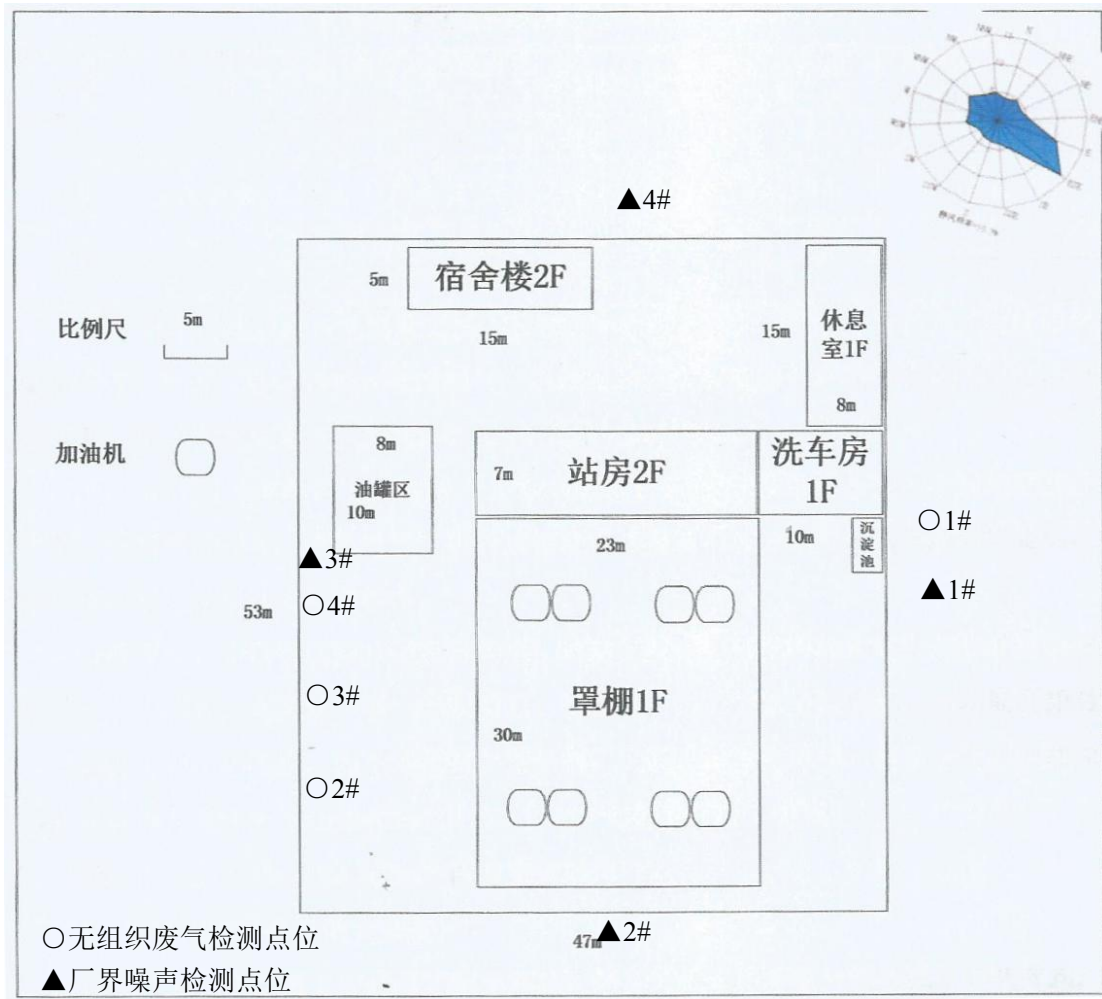
图 7-1 无组织排放及噪声检测点位示意图
