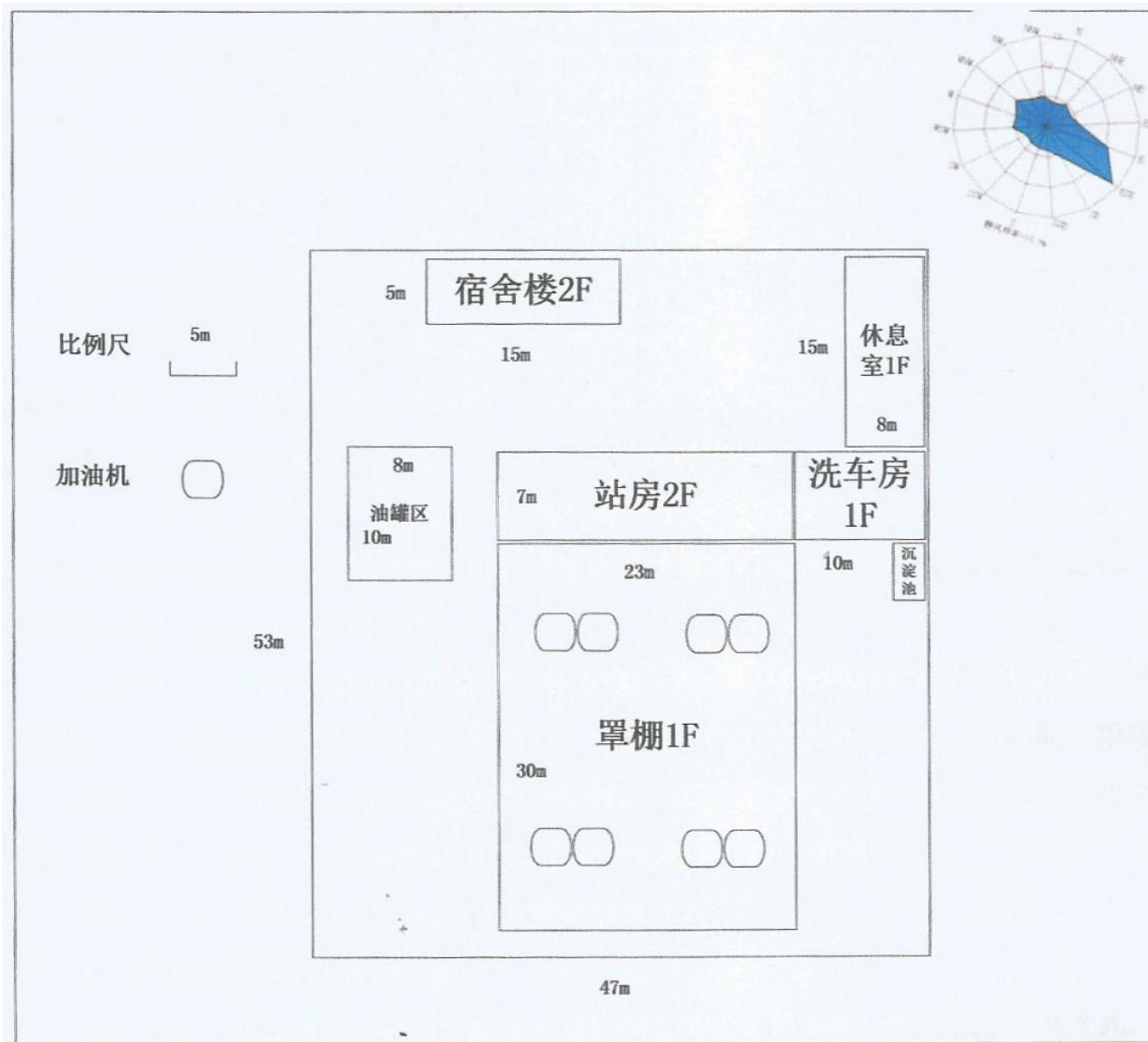
附图 4 厂区平面布置图
