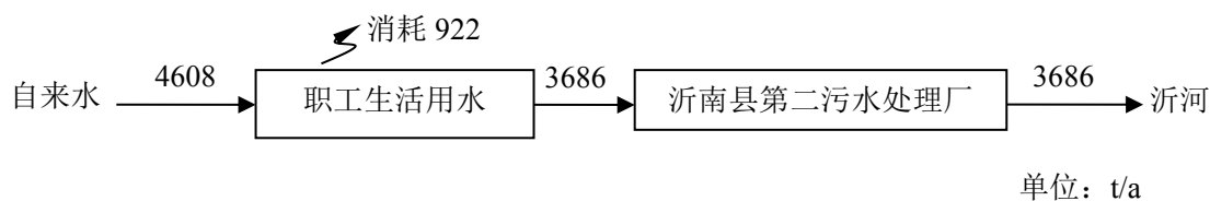
图 3-1 全厂水平衡图
