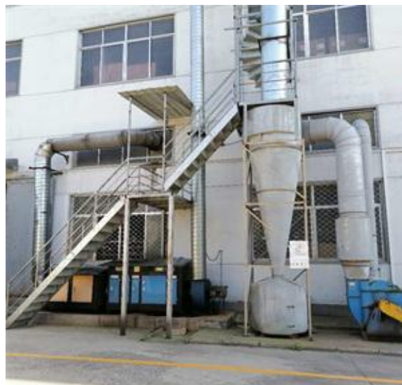
图 4-4 旋风除尘器
