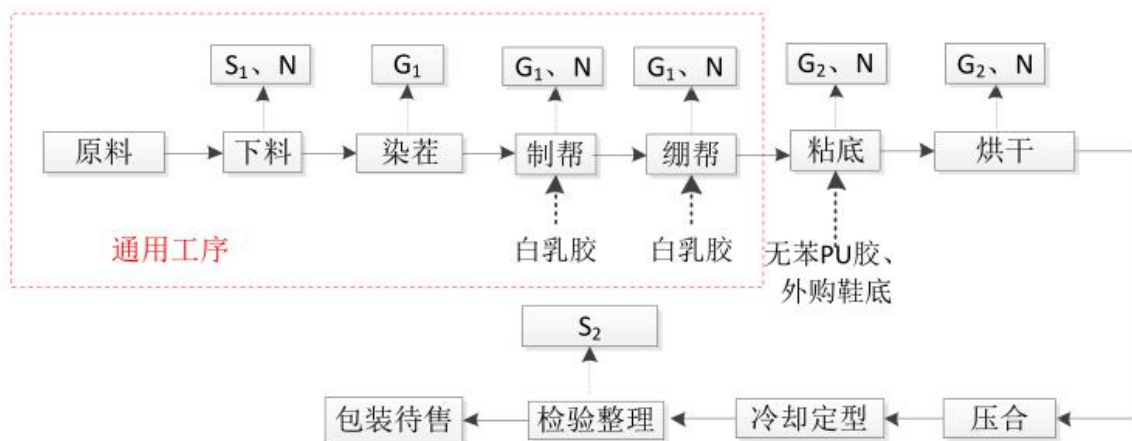
图 3-4 冷粘安全鞋工艺流程及产污环节图
