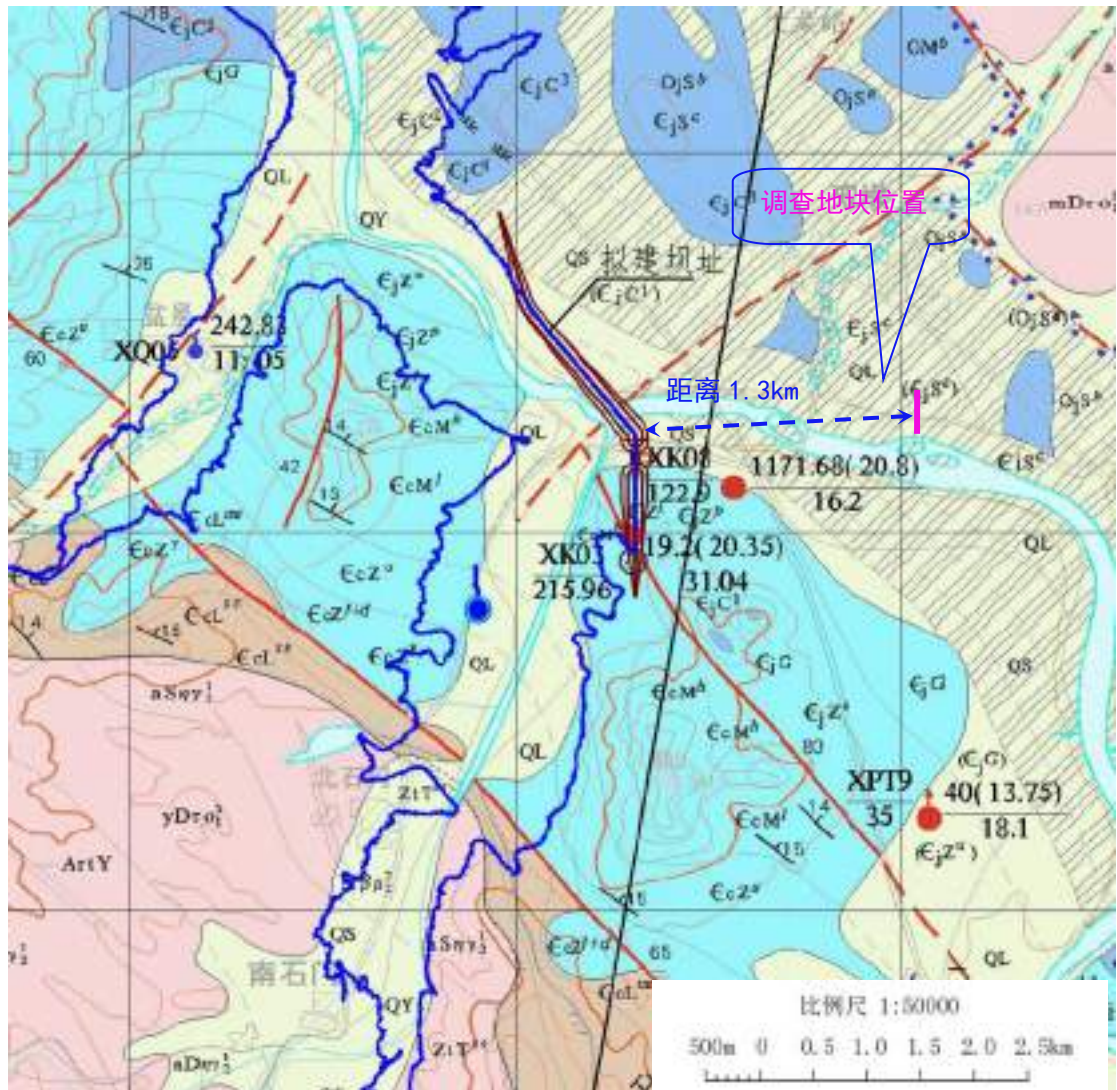
图 3-5 调查地块与大坝相对距离示意图
