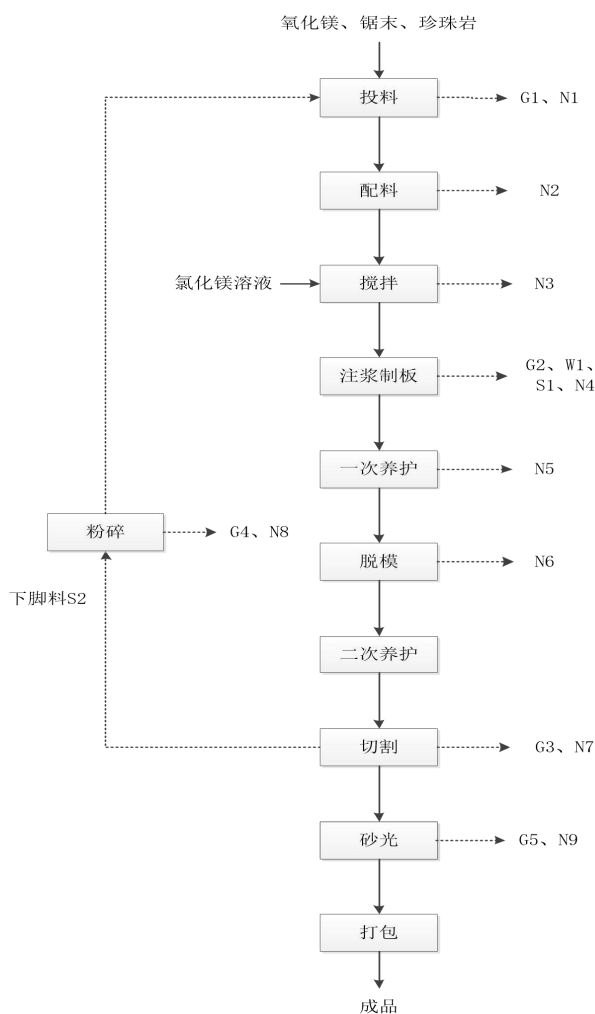
图 4-2 防火板生产工艺流程图
